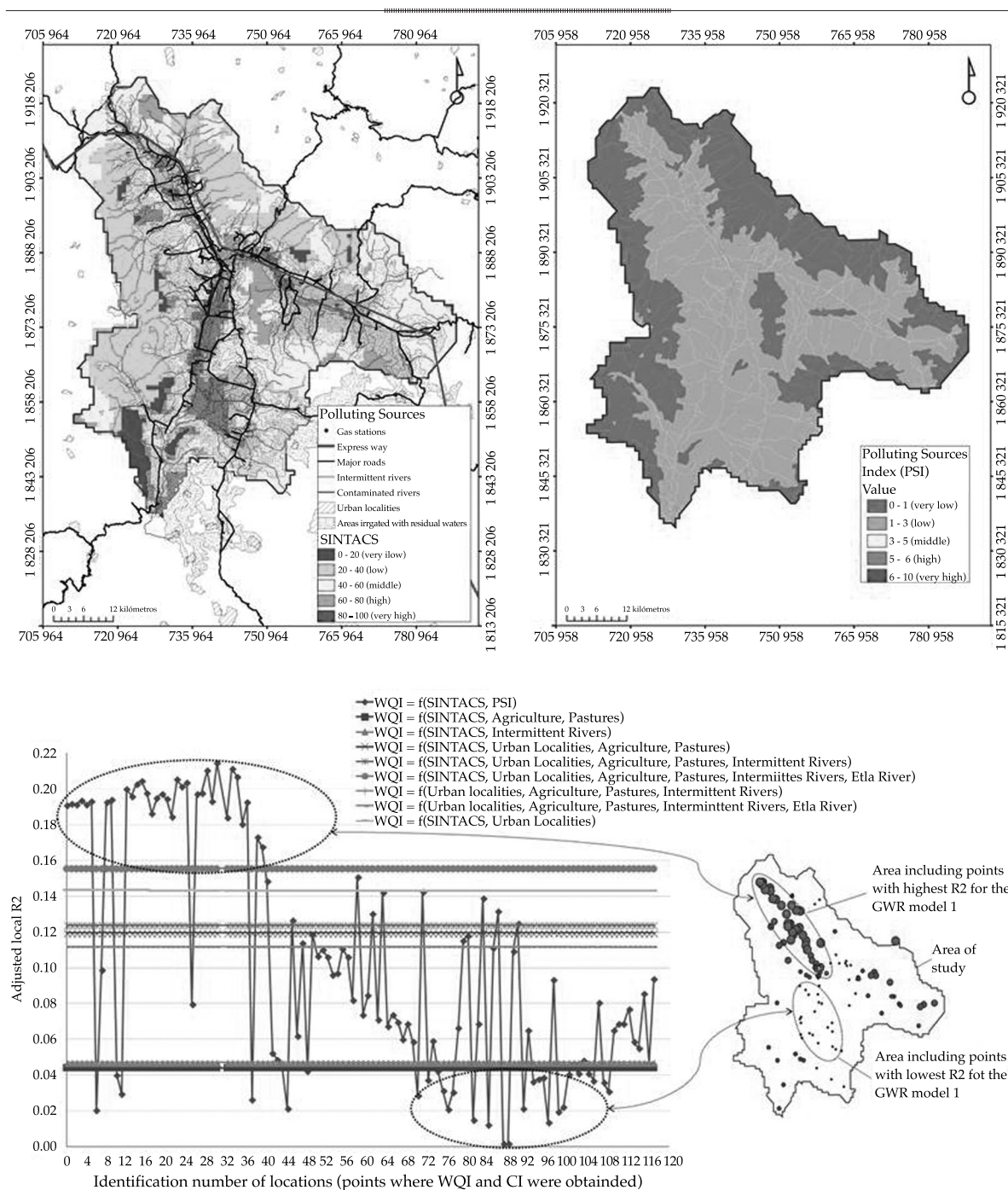
Figura 3. Capas utilizadas para la generación del índice de fuentes de contaminación (PSI), sobre una determinación geográfica del índice SINTACS (arriba izquierda). Especialización de PSI (arriba derecha). Resultados (coeficientes ajustados de correlación local) de la regresión geográficamente pesada (abajo izquierda), así como su distribución espacial en la zona de valles Centrales de Oaxaca, México (abajo derecha) (Ramos-Leal et al. , 2011).
