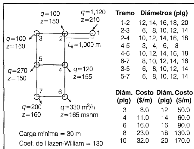
Ilustración 6. Red de Alperovits y Shamir (1977).
