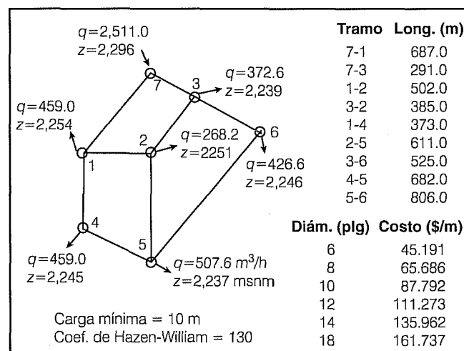
Ilustración 7. Red de Carrillo et al. (1998).
