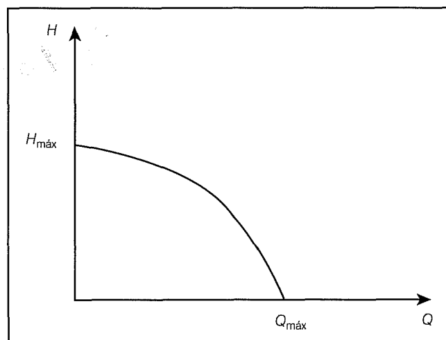
Ilustración 2. Curva característica de una bomba.
